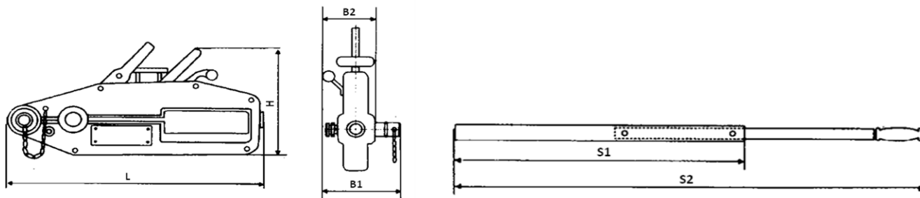
Beispielhaftes Modell
